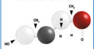
DHEA (Déhydroépiandrostérone)
